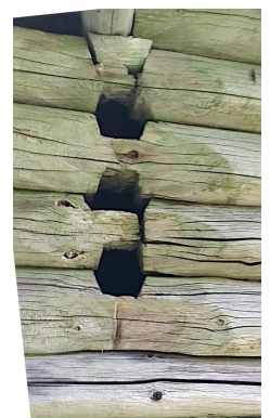
Hålen efter loftgångens vägg i röstet är av samma typ som hörnknutarna.
